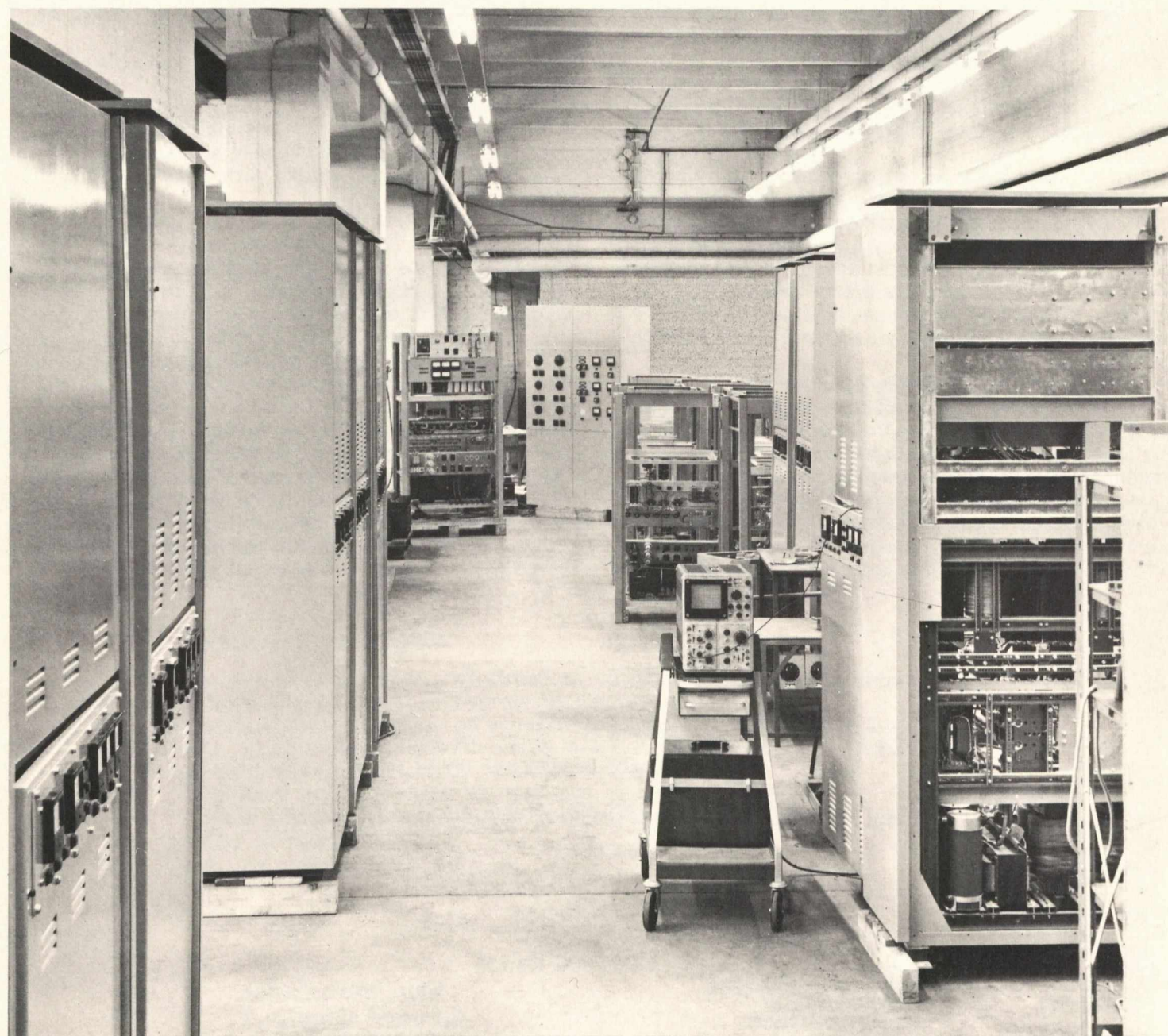
Vaihtosuuntaajia vasemmalla, oikealla tasasuuntaajajärjestelmä. Taustalla lasiuunin mängin ja polttoöljyn suhdesäiliöautomaatiikka.
