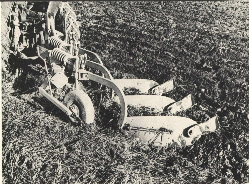
Uusi täysautomaattinen AGROMAT aura, Fiskarsin Konepaja.
