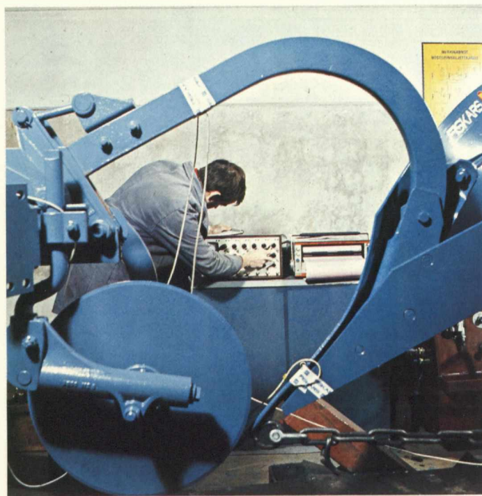
Rauno Ollila testaamassa auran laukaisulaitetta Fiskarsin Konepajalla.
