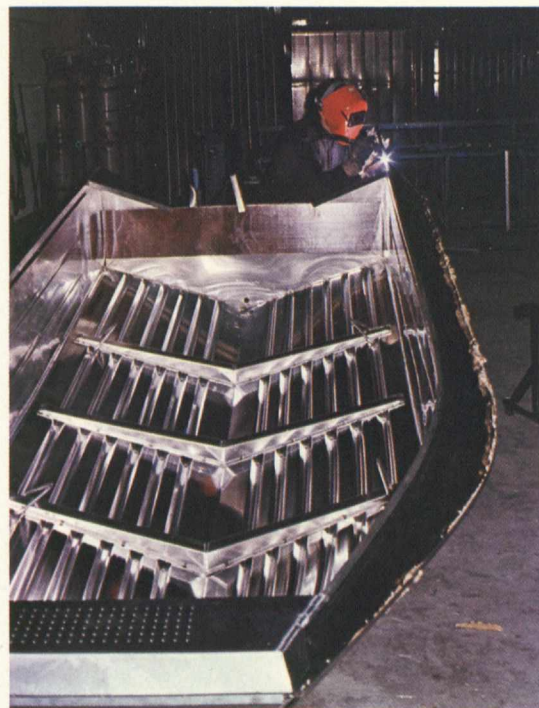
Mauno Leppälä hitsaamassa WorkBusterin peräpeiliä. Kuvaaja: Oiva Järvinen, Inhan tehtaast. Yhtiön valokuvauskilpailussa palkittu kuva.
