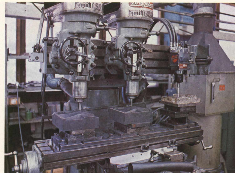
Työkalutehtaalla valmistetaan suuri osa yhtiön eri tehtailla tarvittavista konetyökaluista. Kuvassa jyrsitään elektrodeja, joita käytetään kirveiden teossa tarvittavien työkalujen valmistukseen.
