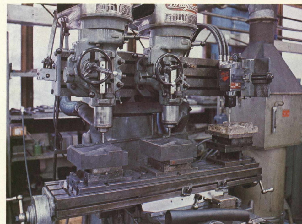
Verktögsfabriken tillverkar en stor del av de maskinverktyg som bolagets fabriker behöver. Här fräses elektroder som användes vid tillverkningen av yxverktyg.
