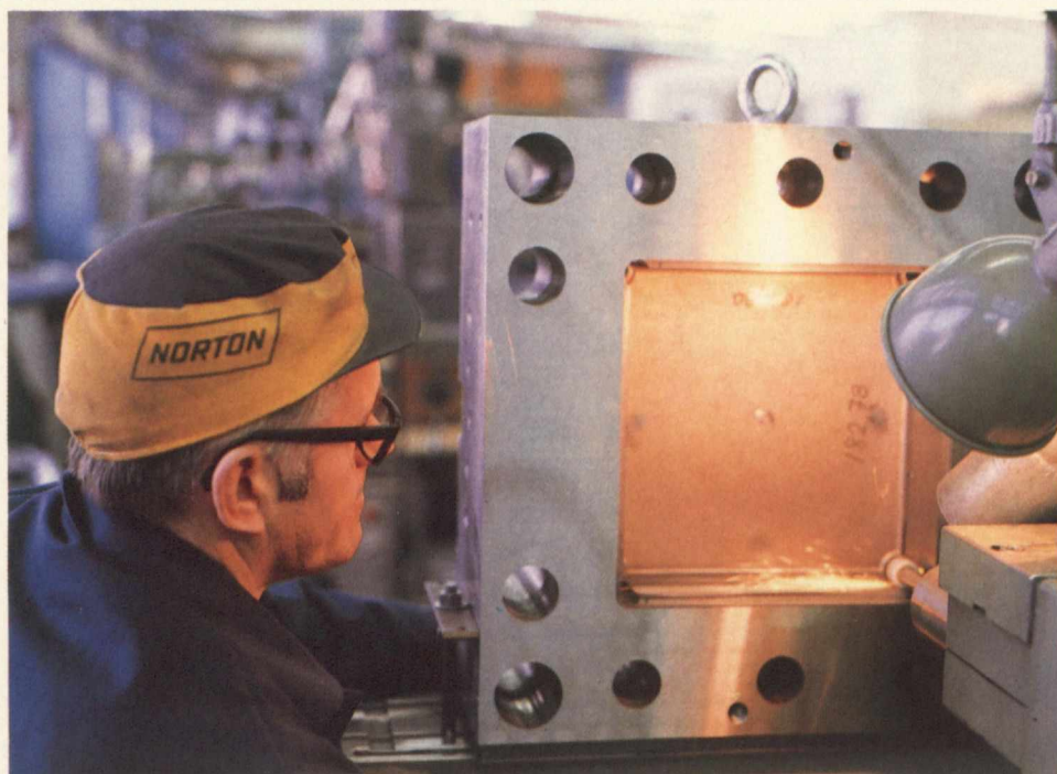
Produktionsverktyget är av avgörande betydelse för produktens slutliga kvalitet. Martti Mäkiranta slipar på Verktygsfabriken ett plastverktyg som behövs vid tillverkningen av lock för EK-kapslingar.
