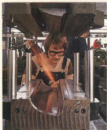
På verktygsfabriken har färdigställt ett verktyg, som används för tillverkning av en plåtdetalj för Sisu lastbilar.
