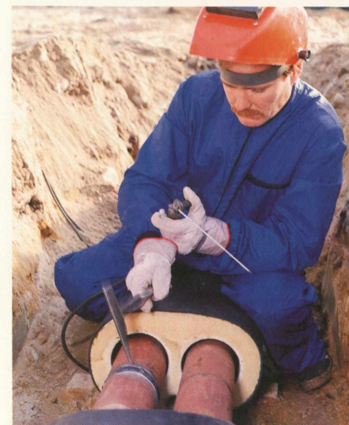
Fiskatherm är ett isoleringssystem för fjärrvärme som spar både energi och arbete. Det förorsakar inga tråkiga överraskningar varken för planeraren eller för montören.
